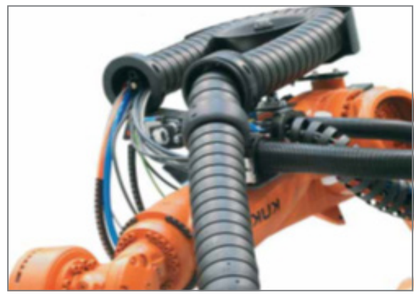
适用于6轴机器人的triflex®RSP系统
