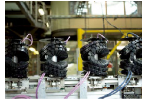
拖链和电缆的扭转测试。
