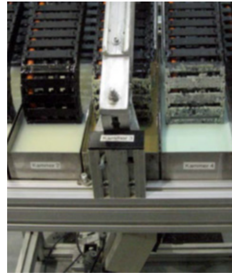
拖链和电缆的扭转测试。
