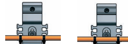
版本 01 - 短接头 short bracket
