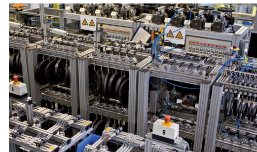
工程塑料轴承技术: 经上千次的测试 ... 模拟真实的环境
